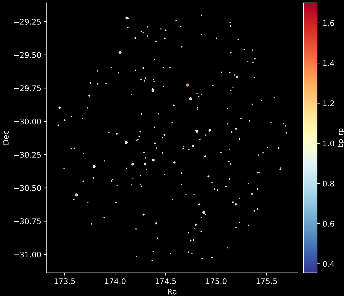
GALAH DR4 Field: [463] Stars: 199
