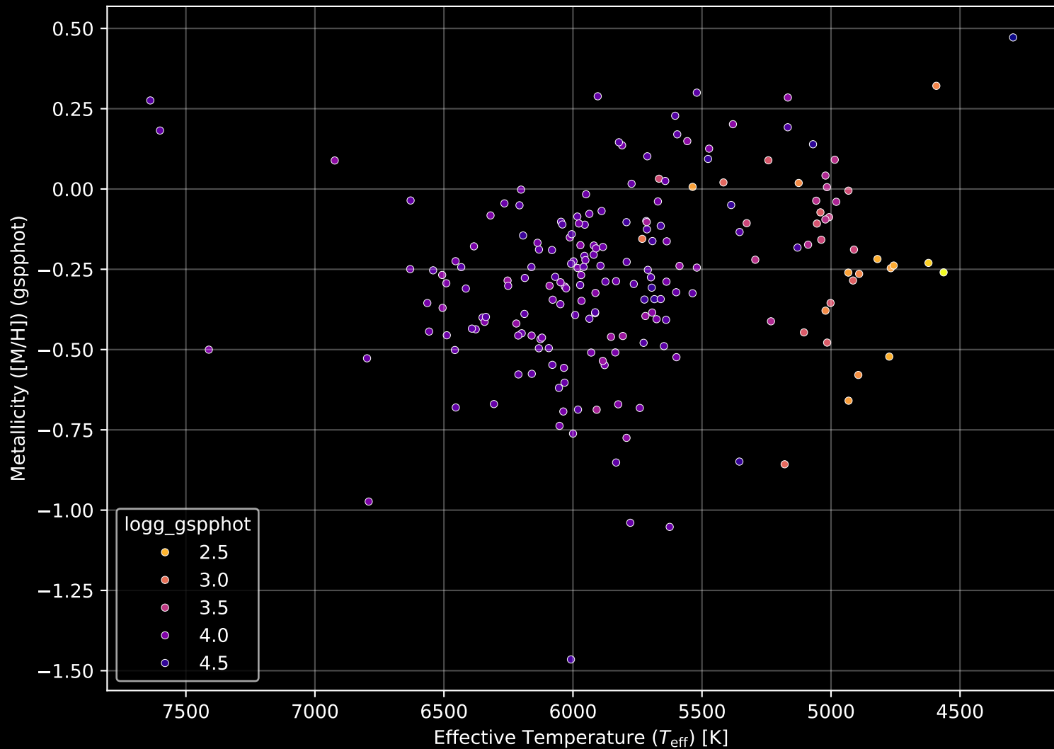
GALAH DR4 Field: [463] Stellar Population Parameters (n= 199)
