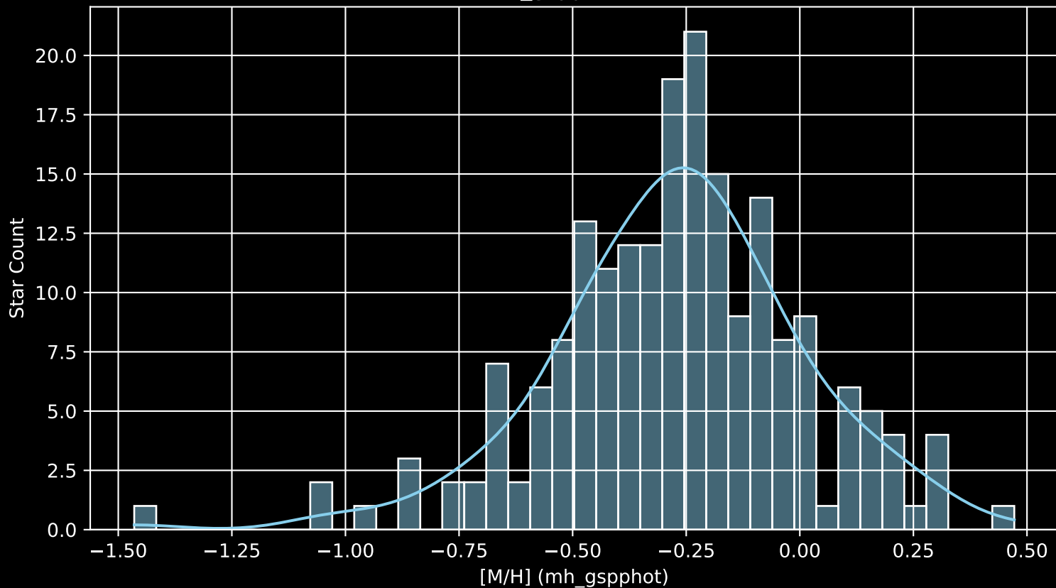
GALAH DR4 Field: [463] [M/H] (mh_gspphot) (n= 199)
