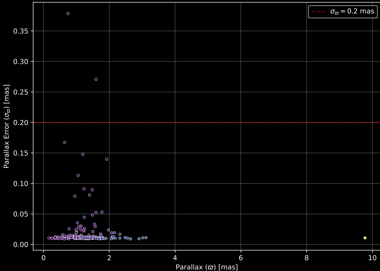
GALAH DR4 Field: [463] Parallax Quality (n= 199)
